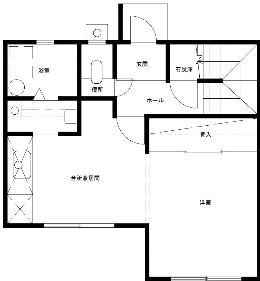
1階平面図
