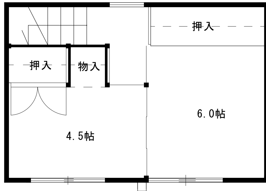
2階平面図
