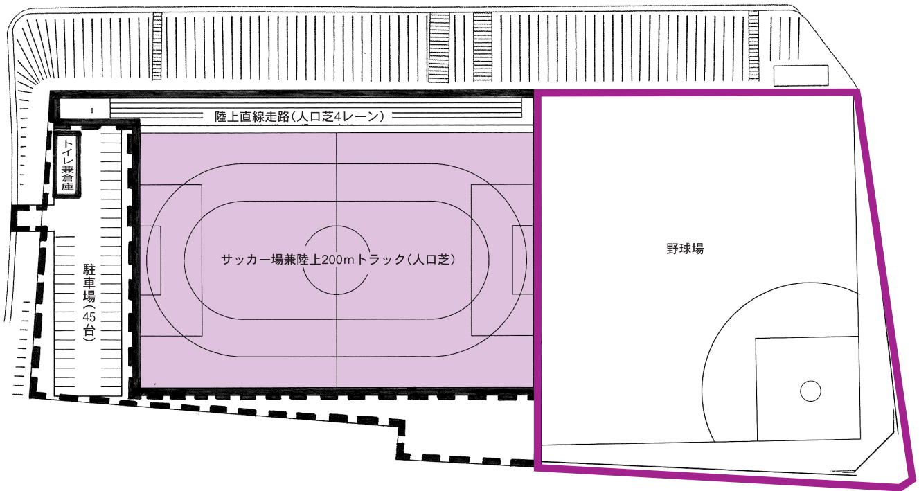
松前中学校グラウンド平面図
